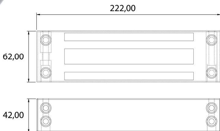
DIMENSIONS VENTOUSE
